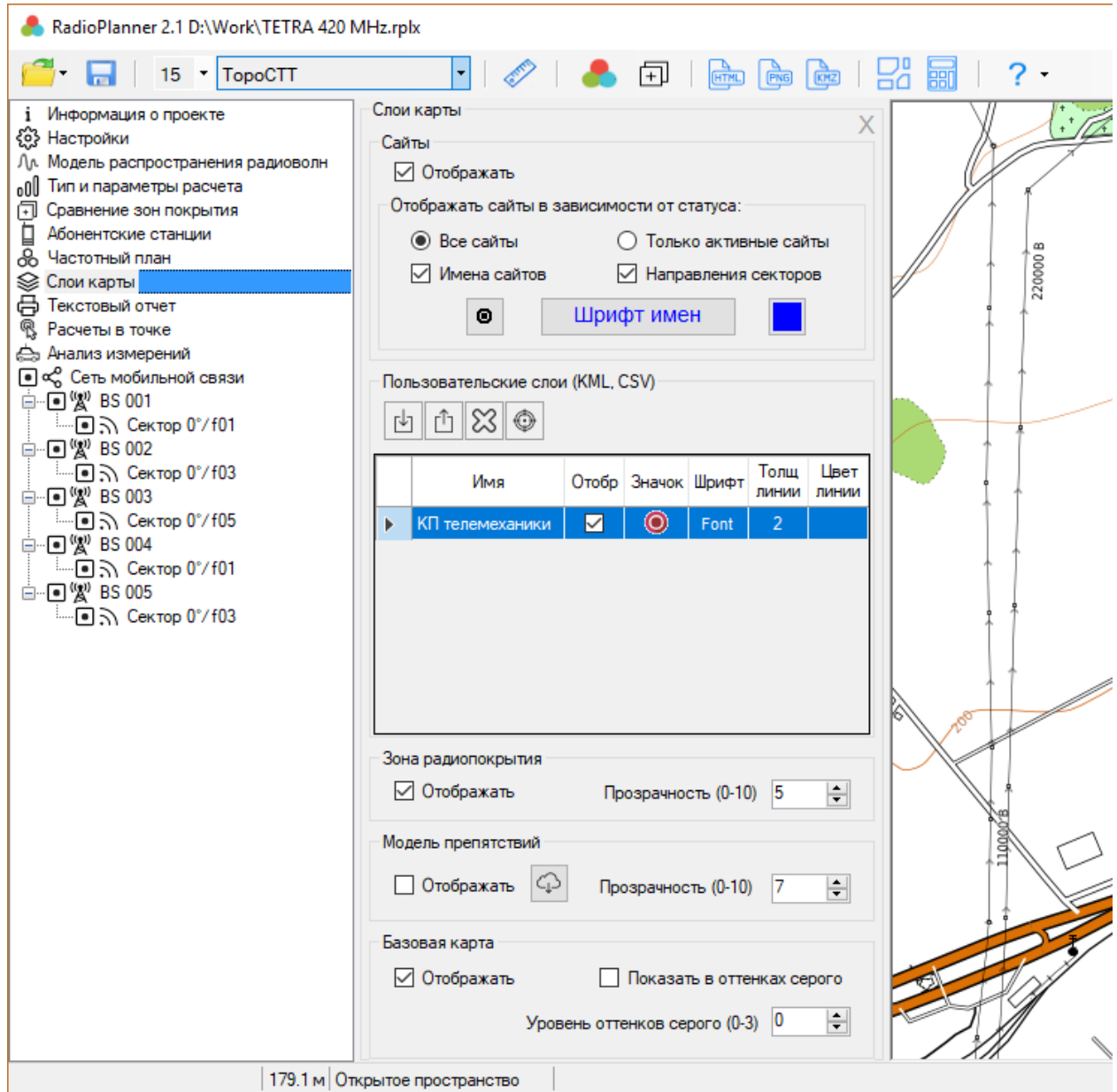
Рисунок 4. Слои карты
