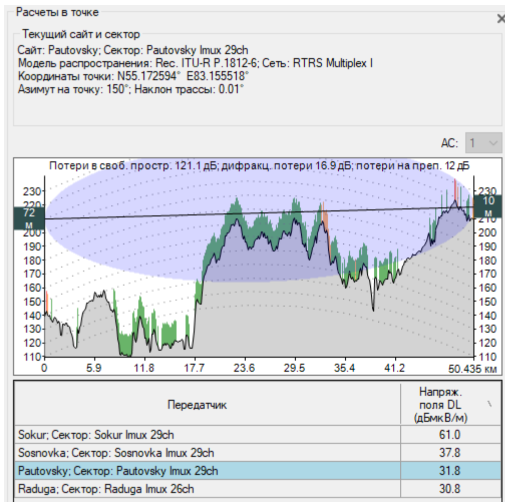
Расчеты в точке для ТВ передатчика
