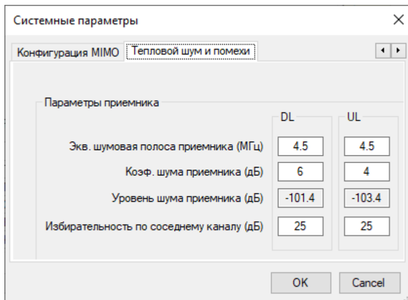
Тепловой шум и помехи для LTE
